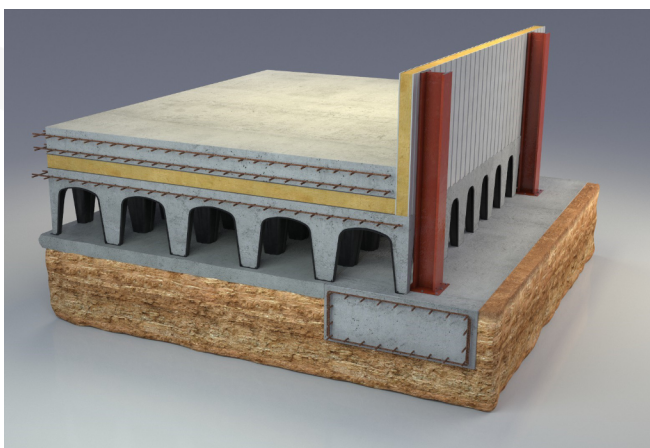
Cámaras frigoríficas
